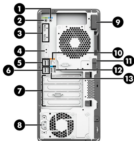
Tabulka 2-4 Součásti na zadní straně věže a jejich popis
